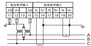
三相三线电流经CT输入 电压直接输入
